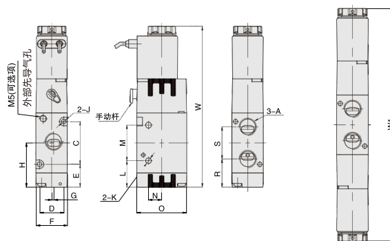
引出线式
