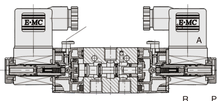
双电控电磁阀
