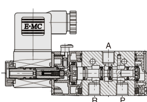
单电控电磁阀（常开）
