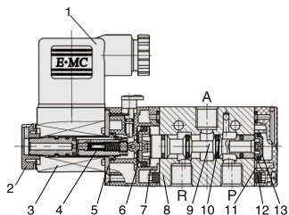
单电控电磁阀（常闭）
